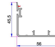
PVC Kanat Ara Bindirme Contası P.A.232.5700.600.0.00.01
