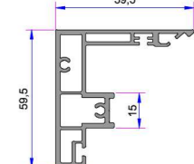
Üç Bölmeli Sürme Alm. Orta Kayıt Profili Profili YENİ Yapılacak
