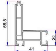
Sineklik Ray Profili P.A.232.5802.600.0.00.19
