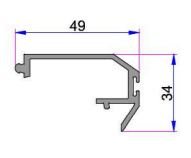
Alm. Kasa Kanal Kapama Profili AD 16 - 013
