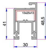
Sürme Sineklik Kanat Profili P.A.242.2305.600.0.00.01
