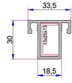
Sürme Sineklik Orta Kayıt Profili P.A.242.3200.600.0.00.01
