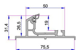
Çift Ray Adaptör Profili P.A.232.5800.600.0.00.19
