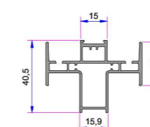
Alm. Kulaklı Çift Kanat Adaptörü Profili YENİ Yapılacak
