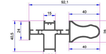
Alm. Griyajlı Çift Kanat Adaptörü Profili YENİ Yapılacak
