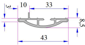
WF-BA-INT043 Battue intérieure de 43 mm Code: P.A.900.6303.600.0.BC.03
