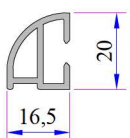
WF-HA-REJ020 Rejet d'eau quart de rond de 20 mm Code: P.A.900.6307.600
