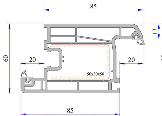
Door Sash Profile
