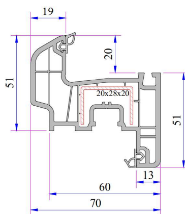
WF-OU-70L051 Ouvrant de 70 mm pour fenêtre
