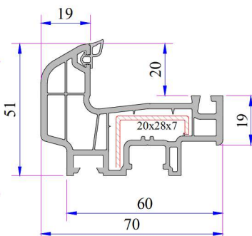
WF-BA-70L051 Battement intégré de 70 pour ouvrant de fenêtre
