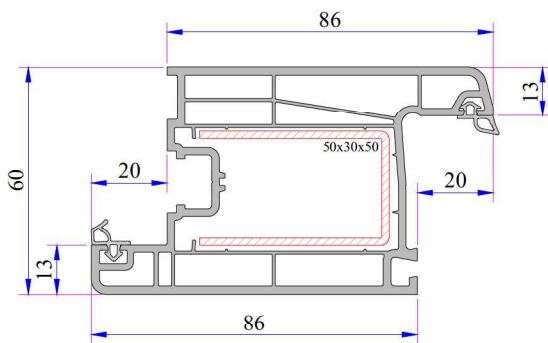
Door Sash Profile
