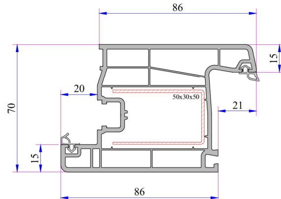
Door Sash Profile
