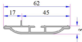
WF-BA-INT062 Battue intérieure de 62 mm sur pour poignée centrée Code: P.A.900.6302.600.0.BC.03
