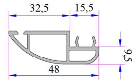
WF-HA-CLAP48 Habillage à clipper 48 mm sur l'aile de 40 mm du dormant Code: P.A.900.6304.600.0.BC.03
