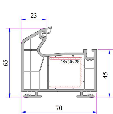
Dormant de base de 70mm largeur
