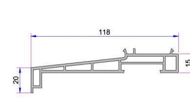
Pervaz Profil P.A.058.5504.600.0.00.19
