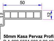
50mm Kasa Pervaz Profil P.A.099.5524.600.0.00.19
