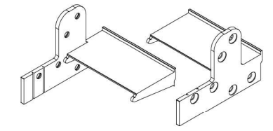
Alüminyum Kasa Eşik Takozu 221013.0000.L - 221013.0000.R
