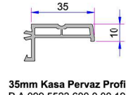
35mm Kasa Pervaz Profil P.A.099.5523.600.0.00.19
