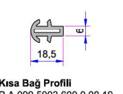
Kısa Bağ Profil P.A.099.5003.600.0.00.19
