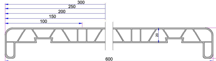
PVC Denizlik Profil (600mm) P.DNZ.01.60.E.600.19
