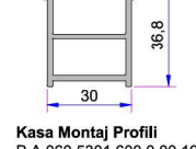
Kasa Montaj Profil P.A.060.5301.600.0.00.19
