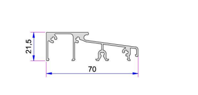
Alüminyum Kapı Eşik Profil AD16-002
