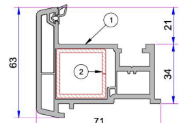
50mm Kasa Pervaz Profil P.A.099.5524.600.0.00.19
