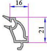
32 mm Dekoratif Contalı Üçlü Cam Çıtası P.A.101.4202.600.0.HC
