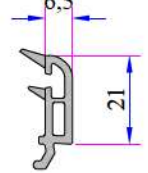
42 mm Contalı Üçlü Cam Çıtası P.A.532.4500.600.0.HC
