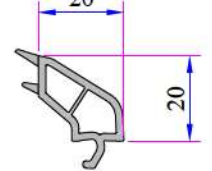
28 mm Contalı Çift Cam Çıtası P.A.101.4100.600.0.HC
