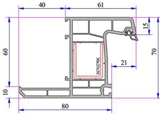
Pervazlı Kasa Profili P.A.750.1200.600.0.BC.01
