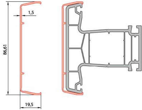
Alüminyum Giydirme Orta Kayıt Profili
