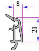
40 mm Contalı Üçlü Cam Çıtası P.A.532.4400.600.0.HC
