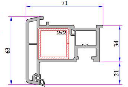
Hareketli Orta Kayıt Profili P.A.750.3100.600.0.BC.19
