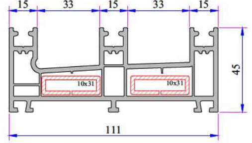
Üç Raylı Kasa Profili P.A.222.1103.600.0.00.01
