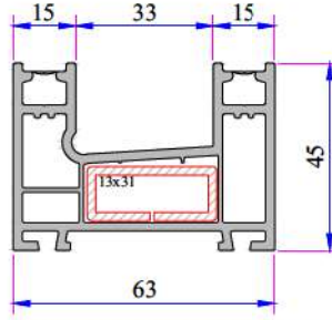
Çift Raylı Kasa Profili (Yeni) P.A.222.1111.600.0.00.01
