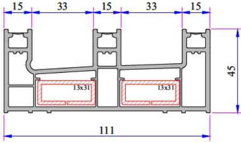
Üç Raylı Kasa Profili (Yeni) P.A.222.1112.600.0.00.01
