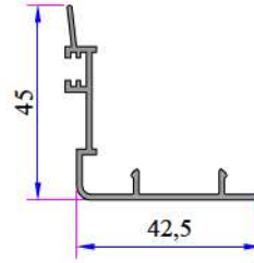
Alm. Süper Kanat Arka Kapama 16032.601.5.1.1.9016
