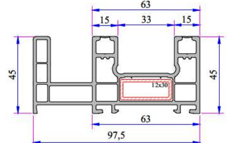
Sürme Sineklik Raylı Kasa Profili P.A.222.1113.600.0.00.01
