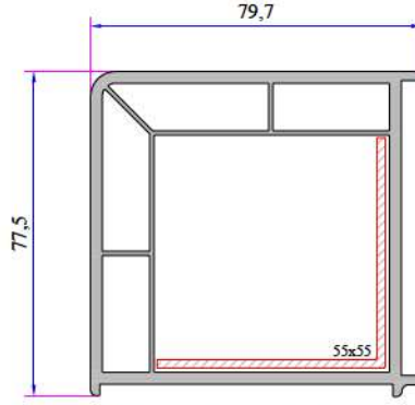
90° Köşe Dönüş Profili P.A.070.5100.600.0.00.19
