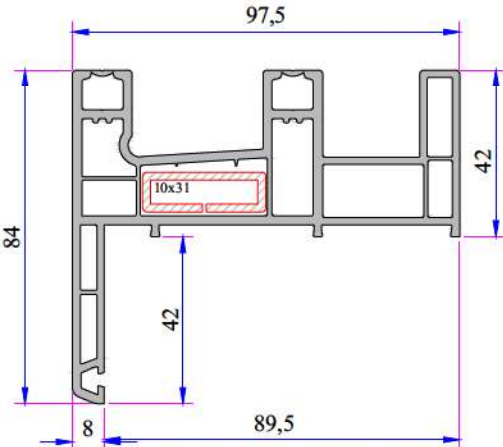
Sürme Pervazlı Sineklik Kasa Profili P.A.222.1109.600.0.00.01
