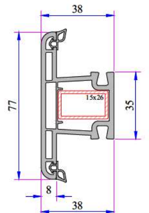
Kanat İçi Orta Kayıt Profili P.A.222.3201.600.0.BC.01
