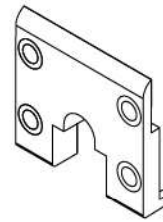
Sürme Kanat Bitiş Parçası 34009-47010
