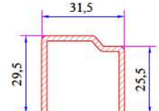
Süper Sürme Kanat Profili Destek Sacı 34022-15027
