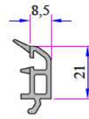
Çift Cam Çıtası 15mm P.A.532.4400.600.0.HC
