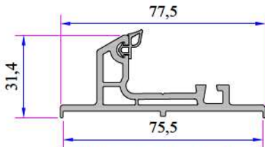
Çift Ray Adaptör Profili P.A.232.5800.600.0.BC.19
