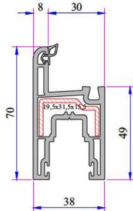
Sürme Kanat Profili P.A.222.2300.600.0.BC.01
