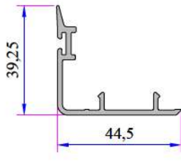
222 Sürme Alın Kapama P.A.222.5708.600
