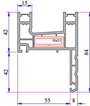
Çift Raylı Pervazlı Kasa Profili P.A.222.1107.600.0.00.01
