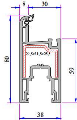
Süper Sürme Kanat Profili P.A.222.2304.600.0.BC.01
