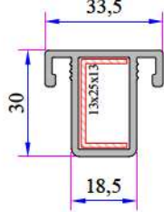
Sineklik Orta Kayıt Profili P.A.242.3200.600.0.00.03
