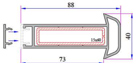
Üniversal Kalın Bağ Profili P.A.058.5000.600.0.19
