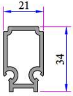
Alm. Çift Ray Adaptörü 16011.601.5.1.1.9016
