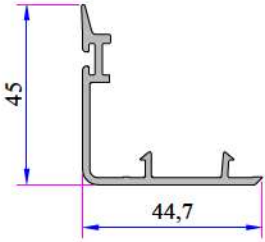
PVC Süper Kanat Arka Kapama P.A.222.5700.600.0.00.19
