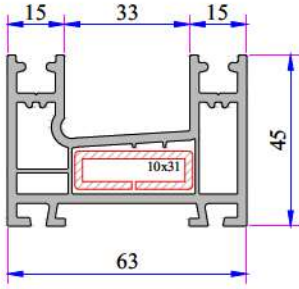
Çift Raylı Kasa Profili P.A.222.1100.600.0.00.01
