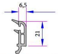
Çift Cam Çıtası 17mm P.A.532.4500.600.0.HC
