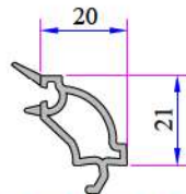
Tek Cam Çıtası 4-6mm P.A.101.4002.600.0.HC
