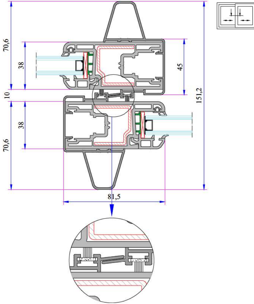
Alm. Çift Ray Adaptörü Montaj Detayı
