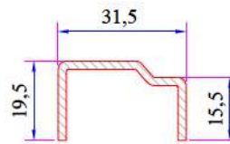
Sürme Kanat Profili Destek Sacı 34022-15026
